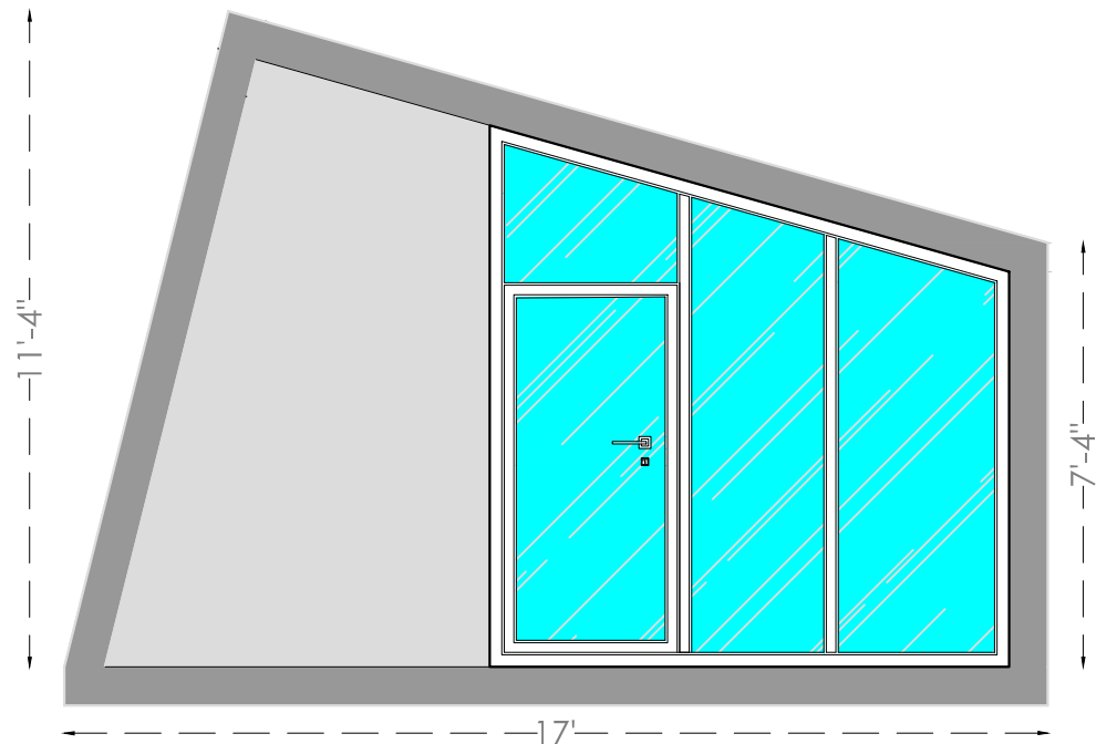
ELEVATION A
