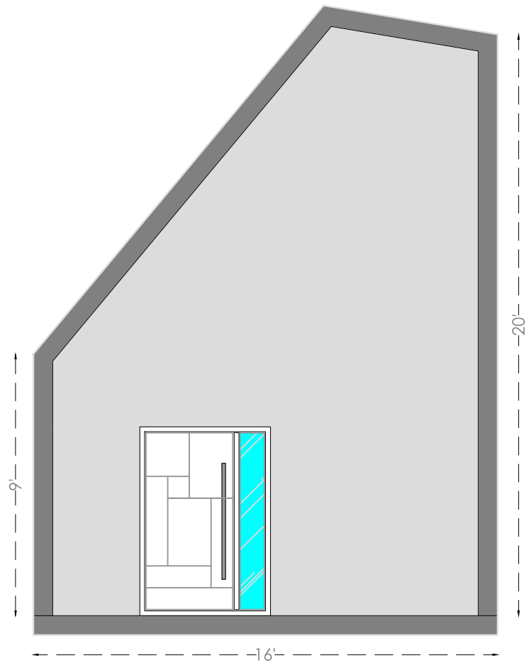
ELEVATION A
