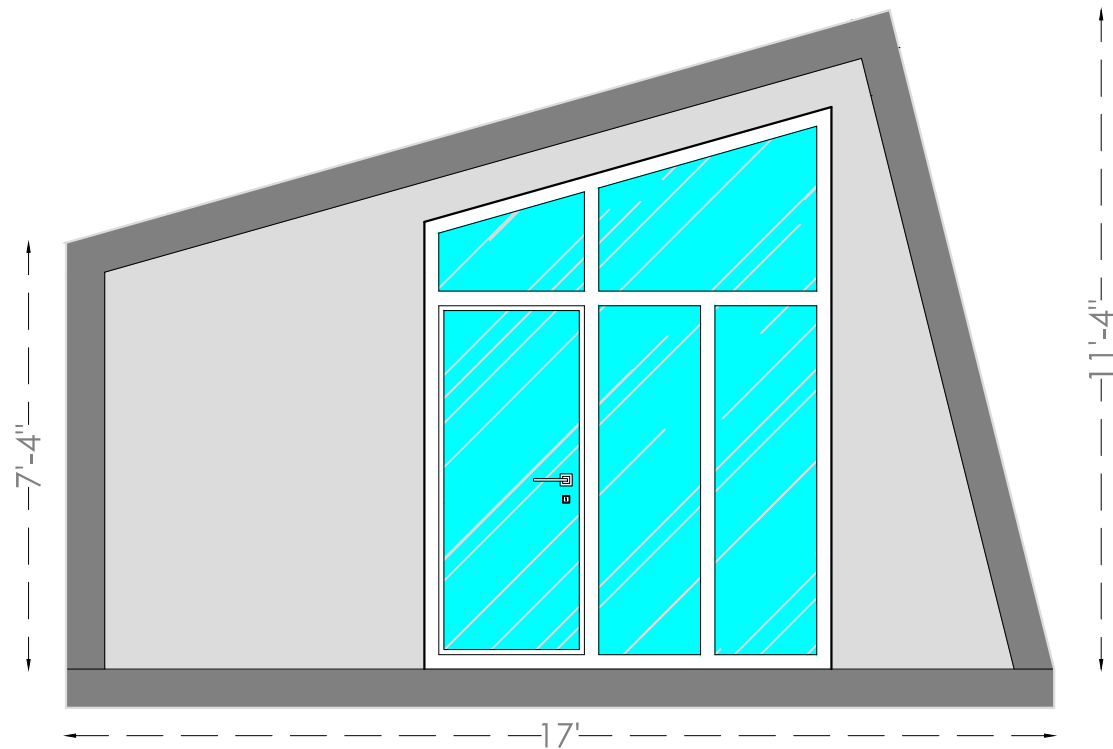
ELEVATION A
